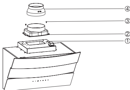
Abb. 3: Abluftstutzen-Teile
